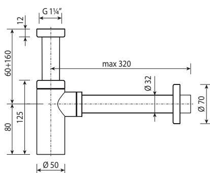
Dekratīvais sifons ir ar hroma apdari un ir ieteicams, ja notekas vieta zem izlietnes ir redzama.
