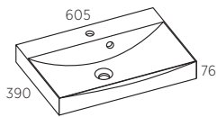
STALVIRŠIS SU INTEGRUOTU PRAUSTUVU 60
