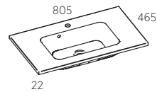
NOVA INTEG PRAUSTUVAS 80
